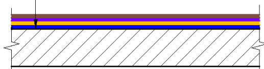
Рис.22. Конструктивный разрез №4.
