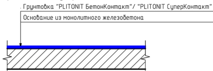
Рис.19. Конструктивный разрез №1.
